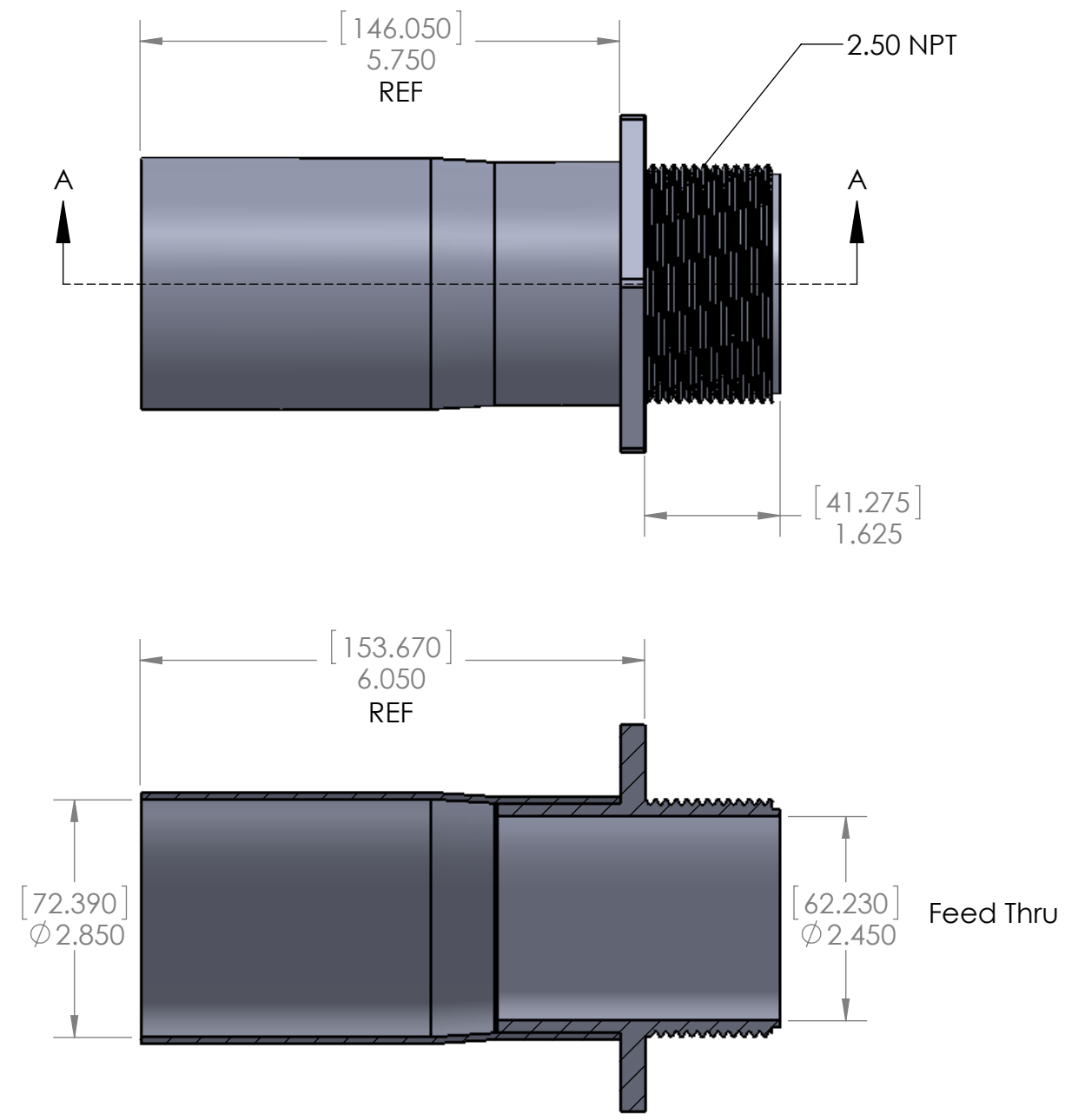
SECTION A-A
