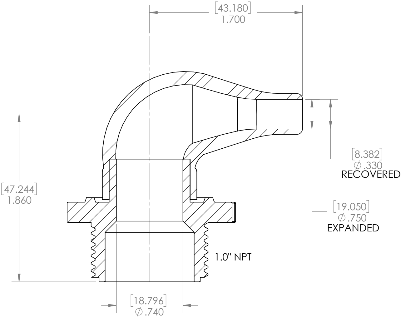
SECTION A-A SCALE 1.5 : 1
